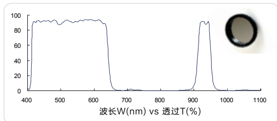
可见红外双带通 940nm (Dual bandpass, FS03-BPD940)
