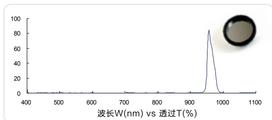
红外带通 950nm (IR bandpass, FS03-BP95020)
