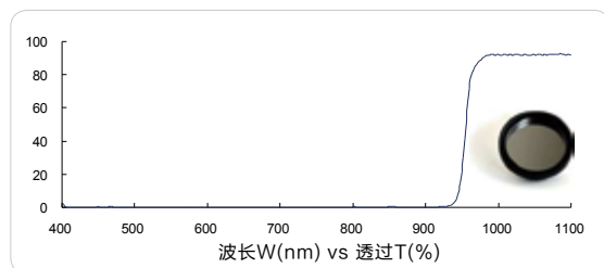
红外长波通 955nm (IR longpass, FS03-LP955)
