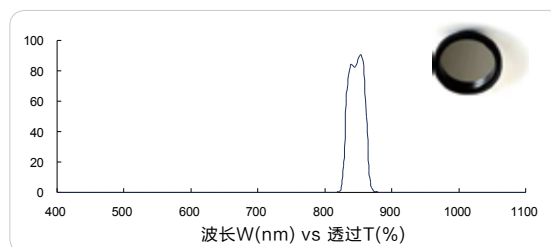
红外带通 850nm (IR bandpass, FS01-BP850)
