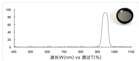
红外带通 940nm (IR bandpass, FS03-BP940)
