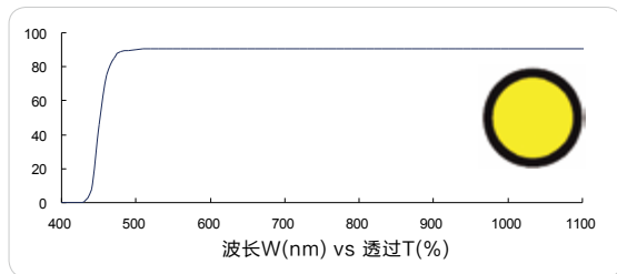
金色长波通 450nm (Violet longpass, FS01-LP450)
