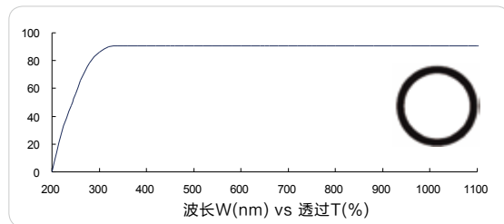
紫外长波通 240nm (UV longpass, FS01-LP240)
