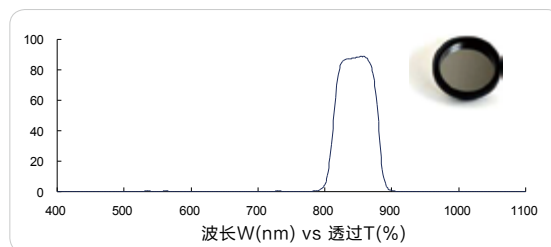
红外带通 850nm (IR bandpass, FS03-BP85070)
