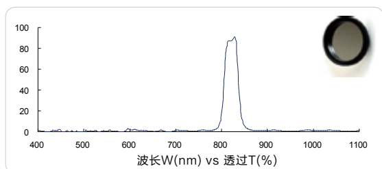
红外带通 830nm (IR bandpass, FS03-BP83030)
