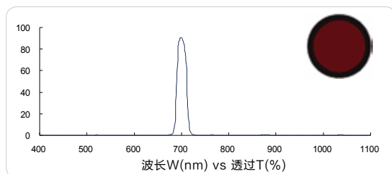
红色带通 700nm (Red bandpass, FS03-BP70020)
