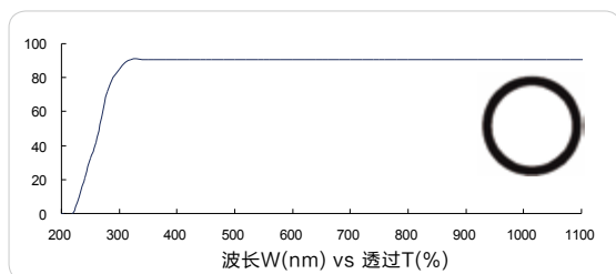
紫外长波通 260nm (UV longpass, FS01-LP260)
