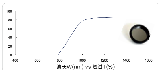
红外长波通 900nm (IR longpass, FS01-LP900)
