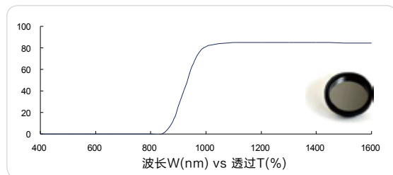
红外长波通 930nm (IR longpass, FS01-LP930)
