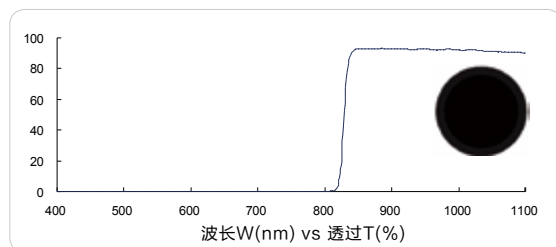
红外长波通 830nm (IR longpass, FS03-LP830)
