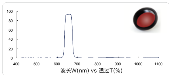
红色带通 660nm (Red bandpass, FS03-BP660)
