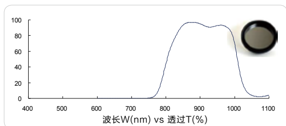
红外带通 850nm (IR bandpass, FS01-BP850206)
