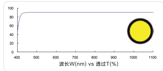
金色长波通 400nm (Violet longpass, FS01-LP400)
