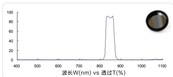
红外带通 850nm (IR bandpass, FS03-BP850)
