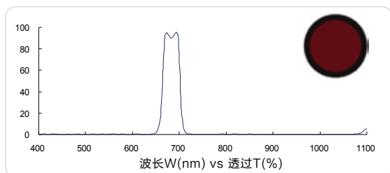
红色带通 690nm (Red bandpass, FS03-BP690)
