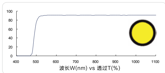
黄色长波通 490nm (Yellow longpass, FS01-LP490)
