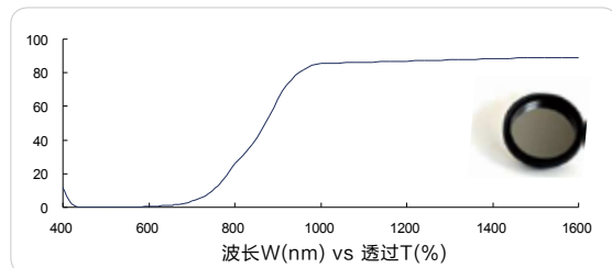
红外长波通 880nm (IR longpass, FS01-LP880)
