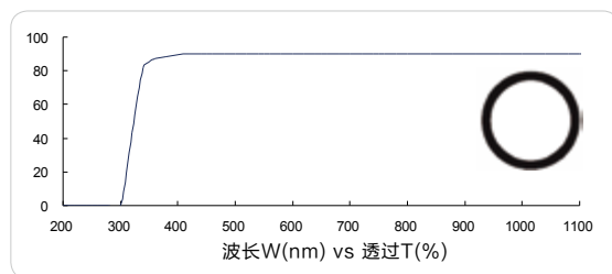
紫外长波通 320nm (UV longpass, FS01-LP320)
