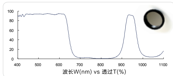
可见红外双带通 940nm (Dual bandpass, FS03-BPD94060)
