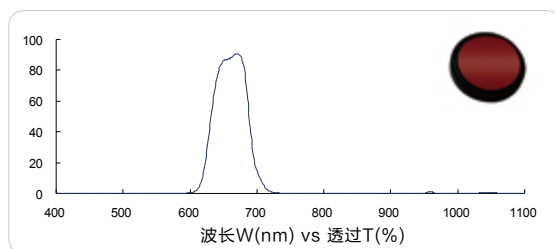
红色带通 660nm (Red bandpass, FS01-BP660)
