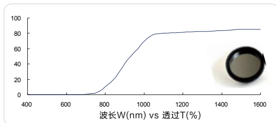
红外长波通 920nm (IR longpass, FS01-LP920)
