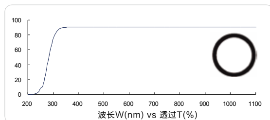
紫外长波通 280nm (UV longpass, FS01-LP280)
