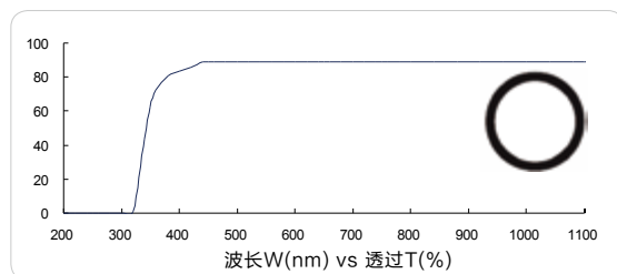
紫外长波通 340nm (UV longpass, FS01-LP340)
