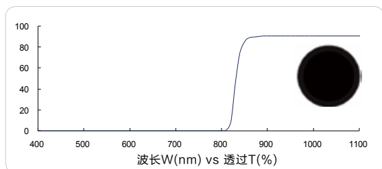
红外长波通 830nm (IR longpass, FS01-LP830)
