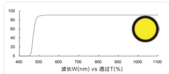
黄色长波通 470nm (Yellow longpass, FS01-LP470)
