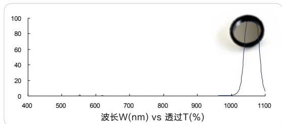
红外带通 1060nm (IR bandpass, FS03-BP106050)
