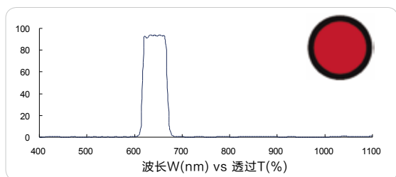
红色带通 650nm (Red bandpass, FS03-BP65050)
