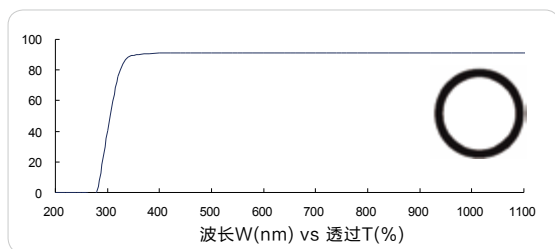
紫外长波通 300nm (UV longpass, FS01-LP300)
