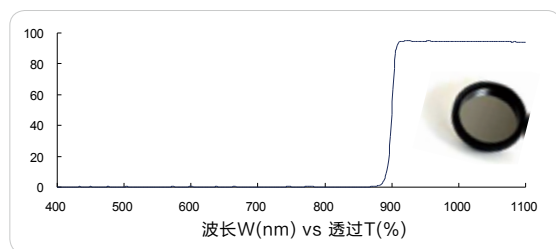
红外长波通 900nm (IR longpass, FS03-LP900)
