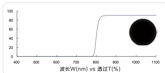
红外长波通 800nm (IR longpass, FS01-LP800)
