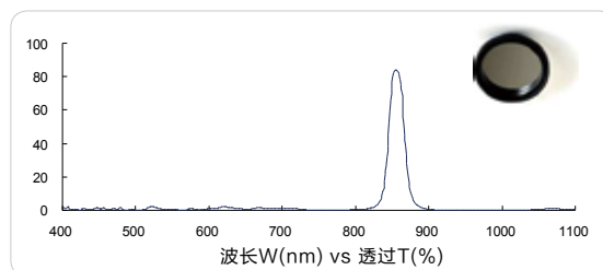
红外带通 850nm (IR bandpass, FS03-BP85020)
